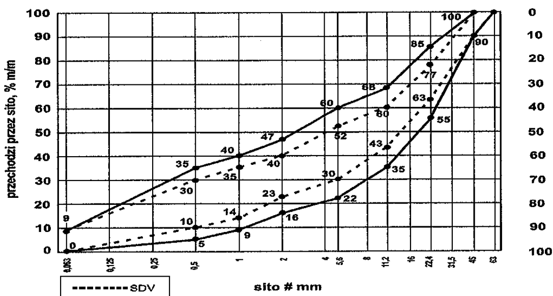
Rys. 2. Krzywe graniczne uziarnienia mieszanki kruszywa niezwiązanego 0/45 mm podbudowy zasadniczej
